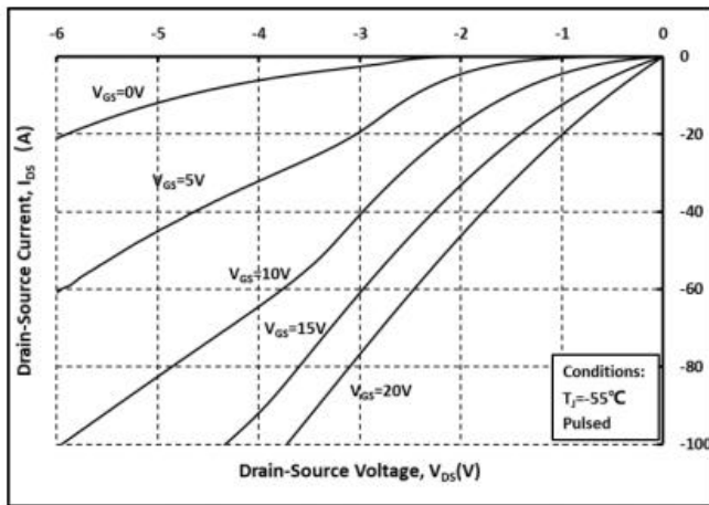
图. 13 第三象限曲线 @ T_j = -55^\circ\text{C}
