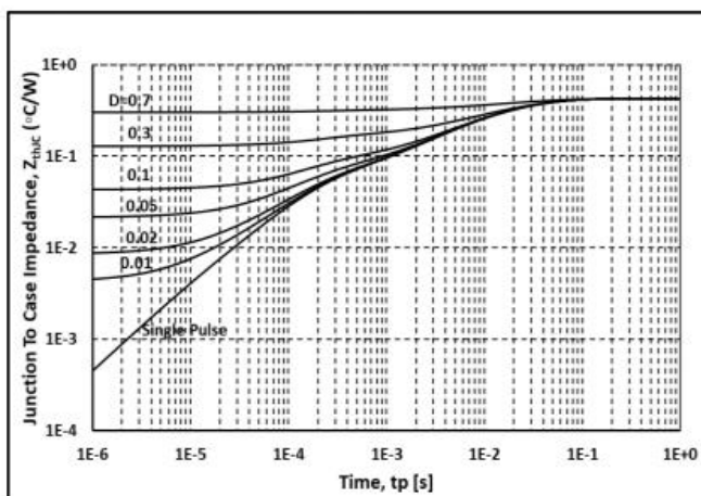
图. 23 热阻曲线
