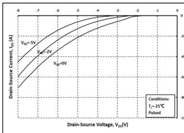
图. 11 体二极管导通曲线 @ T_j = 25°C
